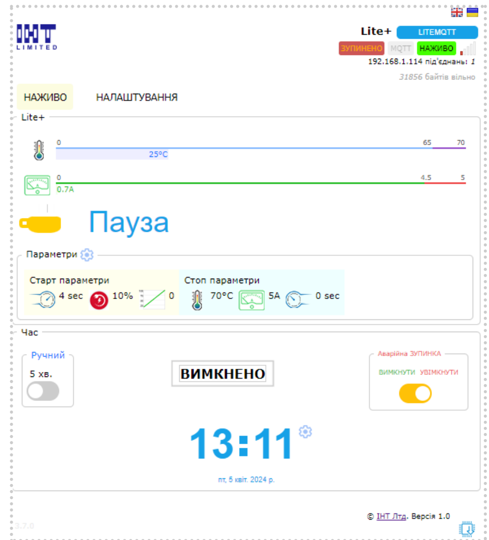
мал. 7 Перша сторінка у повнофункціональному режимі
