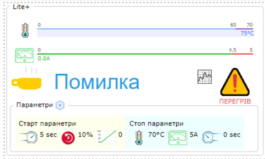
мал. 12 Плитка відображення стану та основних налаштувань ПМП
