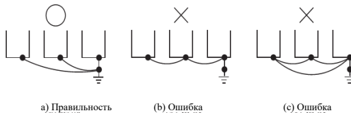
Рис. 4-3 Схема заземления
