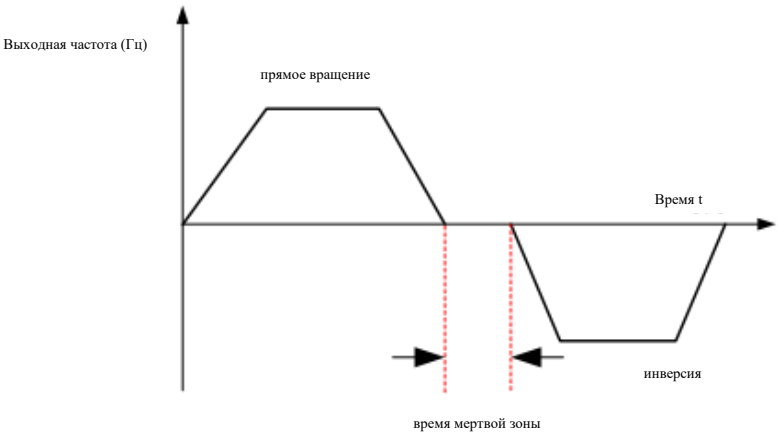
Рис. 7-21 Схема времени прямой и обратной мертвой зоны
