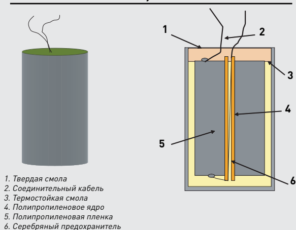
Катушка
