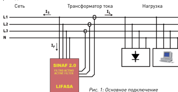
Рис. 1: Основное подключение
