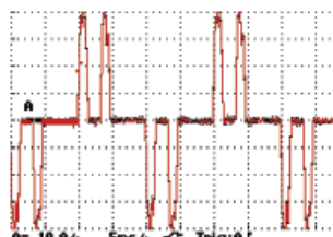
Входной преобразователь без фильтра
