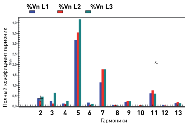
Прием анализа полного коэффициента гармоник
