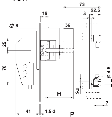
VC1P
