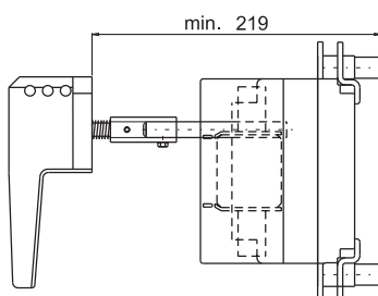
Прямая ручка
