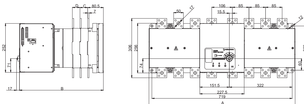
CO5 800 ÷ 3150 A
