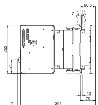
CO6 2000 A
