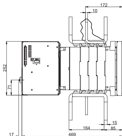
CO6 3150 A
