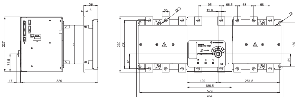
CO4
