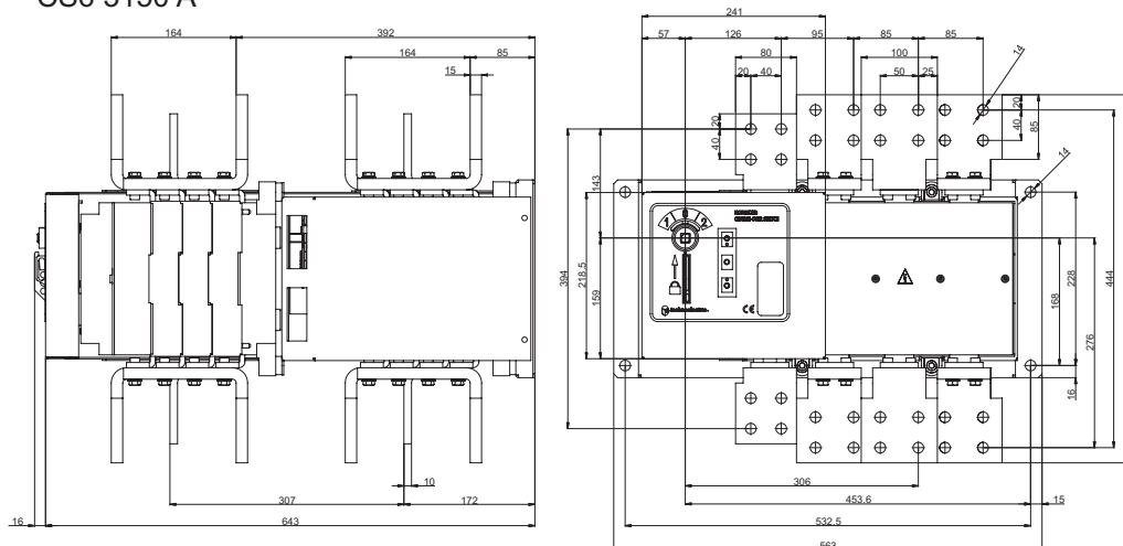
CS6 3150 A
