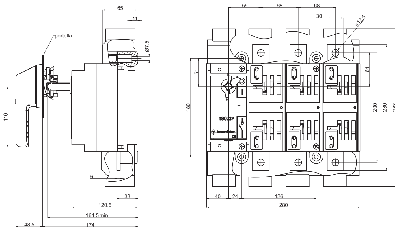
TS073P
