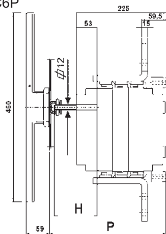
Прямая ручка
