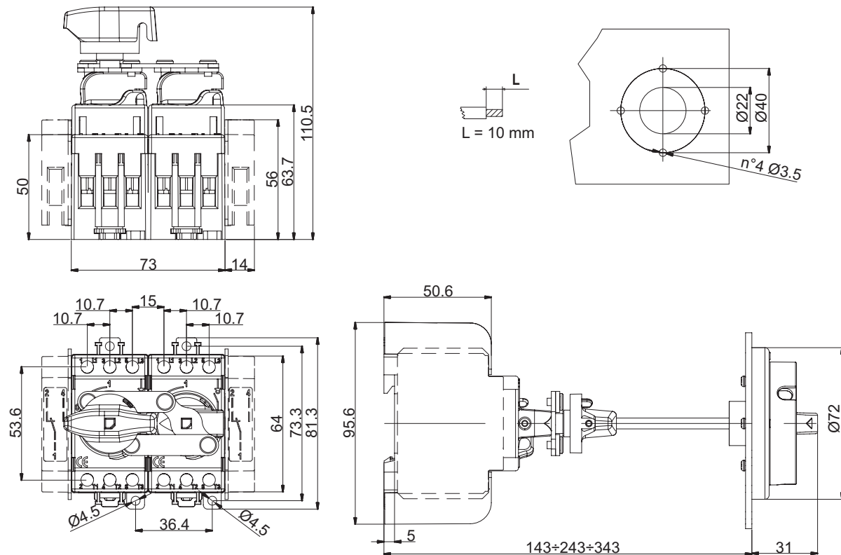
TS016M
