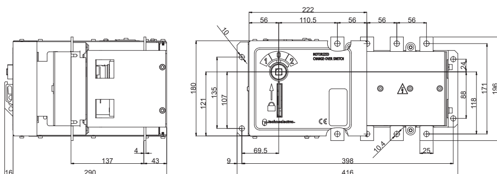
CS3
