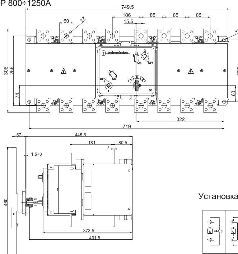
BYP 5P 800÷1250A
