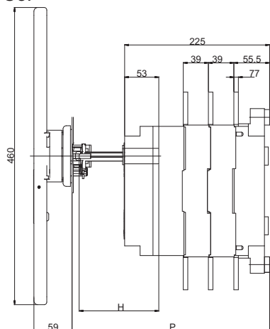
Прямая ручка
