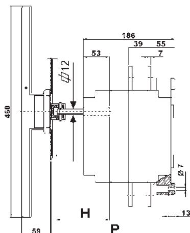
Прямая ручка
