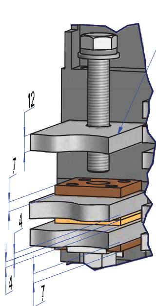
D (0,45 : 1)
