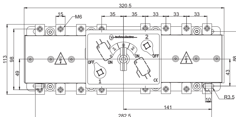
BYP 1P 32 ÷ 160 A
