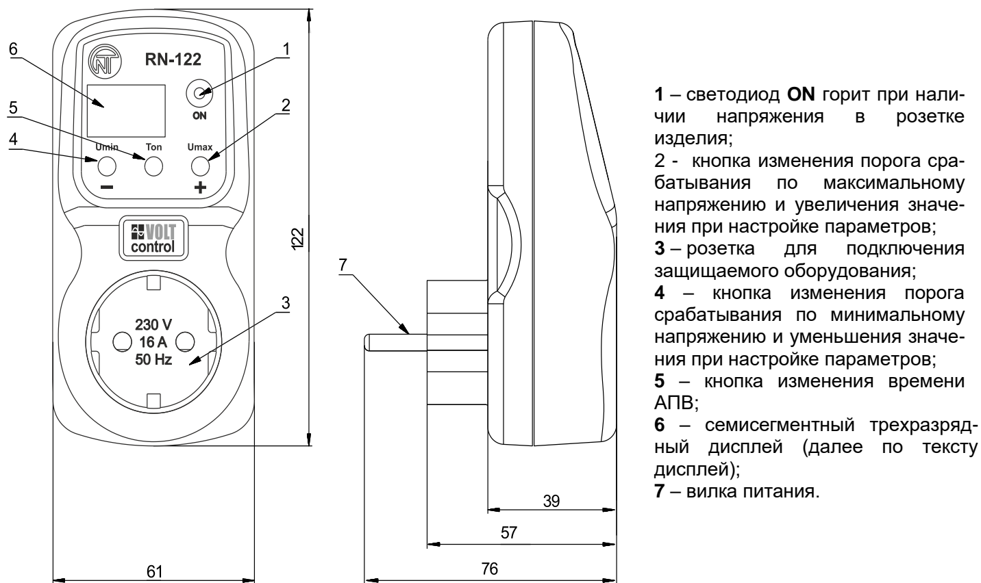
Рисунок 1 – Органы управления и габаритные размеры RN-122
